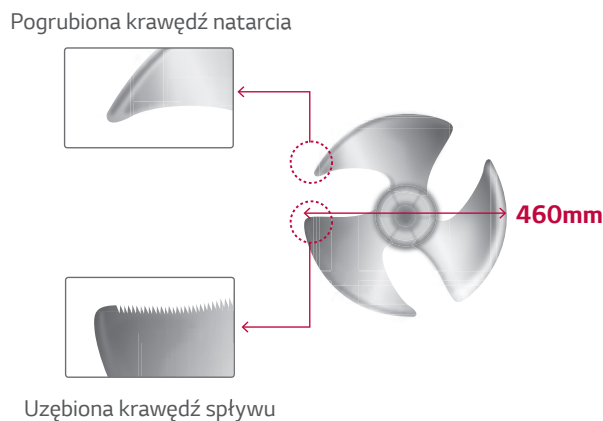
Wentylator typu 2
